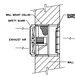
9 WALL FAN DETAIL NTS
